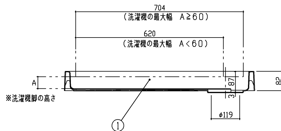
断面A-A
